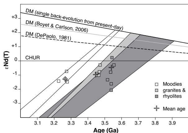
Figure 11 : les âges modèles Sm-Nd des granites et rhyolites du Groupe de Moodies suggère que le protolith de leur source date de 3.8-3.9 milliards d'années. D'après Sanchez-Garrido [thèse, 2012].
