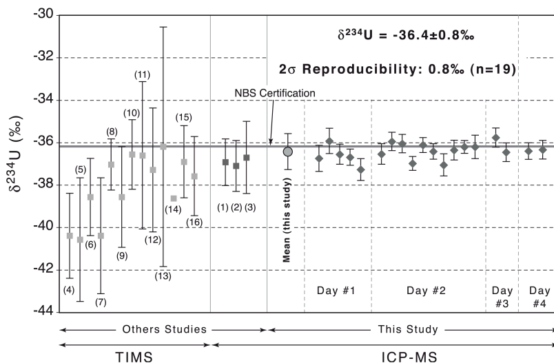
Figure 22 : Gain de précision obtenu lors du développement de l'analyse des rapports isotopiques d'uranium par spectrométrie de masse à source plasma, multi-collecteur (ICP-MS). D'après Deschamps et al. [2003].
