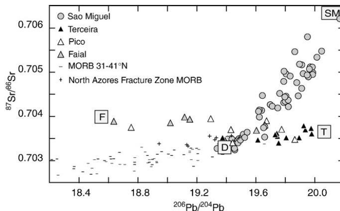
Figure 5 - Variations des compositions isotopiques de Pb et Sr à l'échelle de l'archipel des Açores et définition des pôles de mélange São Miguel (SM), Terceira (T), Faial-Pico (F) et MORB (D) [Millet et al. , 2009].
