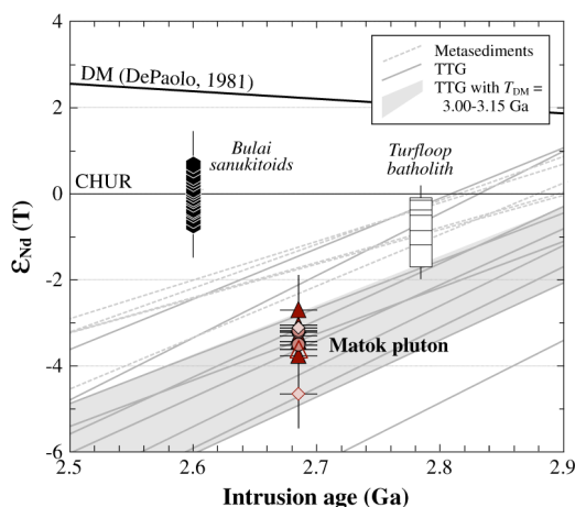
Figure 10 : Rapport isotopique de Nd initial (exprimé en notation \epsilon ) en fonction de l'âge. Les sanukitoïdes s.s. montrent des signatures juvéniles alors que celles des sanukitoïdes marginaux et des granites contemporains sont intermédiaires entre juvéniles et recyclées, en accord avec les modèles pétrogénétiques basés sur les éléments majeurs et en traces. D'après Laurent et al. [2014a].
