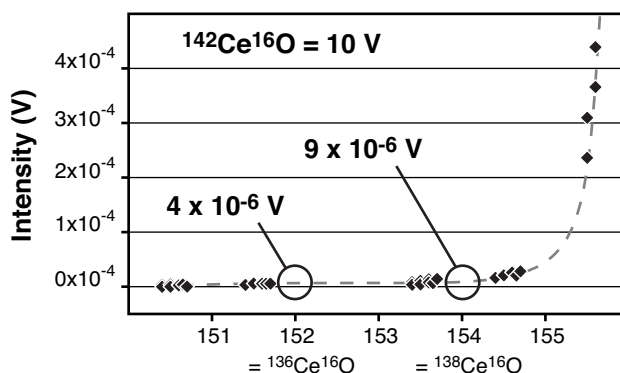
Figure 21 : Forme du pic majeur de Ce ( ^{140}\text{Ce} = \sim 80\text{ V} ) du côté des basses masses, et interférences sur les masses mineures ^{136}\text{Ce} et ^{138}\text{Ce} . A noter que les masses de Ce sont mesurées sous forme oxyde. Modifié d'après Bellot et al. [2015].
