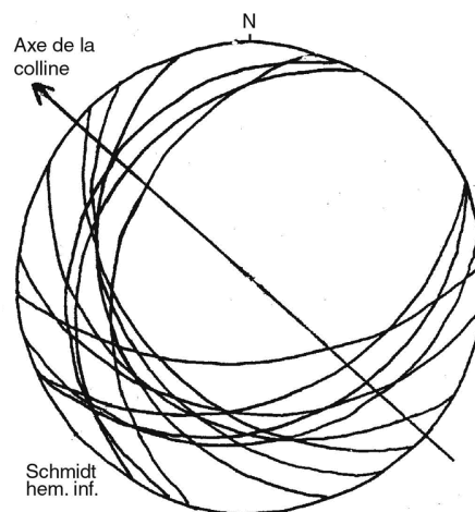
FIG. 5. – Stéréogramme des fractures relevées sur une ride de l'unité bréchique Br III, en amont du Cap La Houssaye. Sur cette station de mesure des plans de fracture, effectuée sur le flanc sud-ouest d'une ride d'allongement général SE-NW dans l'axe du Cap La Houssaye, apparaissent nettement deux familles de plans. La première famille, d'orientation globale NE-SW, à pendage NW ou SE (plans antithétiques), est perpendiculaire à la ride et correspond à son tassement dans l'axe du mouvement. La deuxième famille, d'orientation NW-SE, à pendage systématique SW, dans le même sens que la pente de la ride dans ce secteur, est interprétée comme un ensemble de failles listriques gravitaires.
