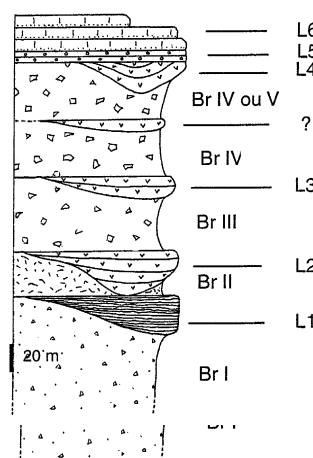
FIG. 4. – Colonne lithologique des unités bréchiques (Br I à Br IV) et des laves interstratifiées (L1 à L6) dans la région du Cap La Houssaye. L1 : coulée de basalte à olivine de type « pahoehoe », L2 à L4 : basalte picritique et basalte à olivine, L5 : basalte plagioclasiq, L6 : mugéarite.
