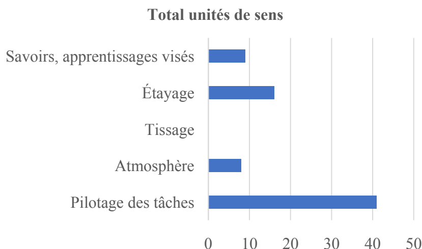
Figure 5. Distribution des unités de sens en fonction des macro-préoccupations enchâssées
