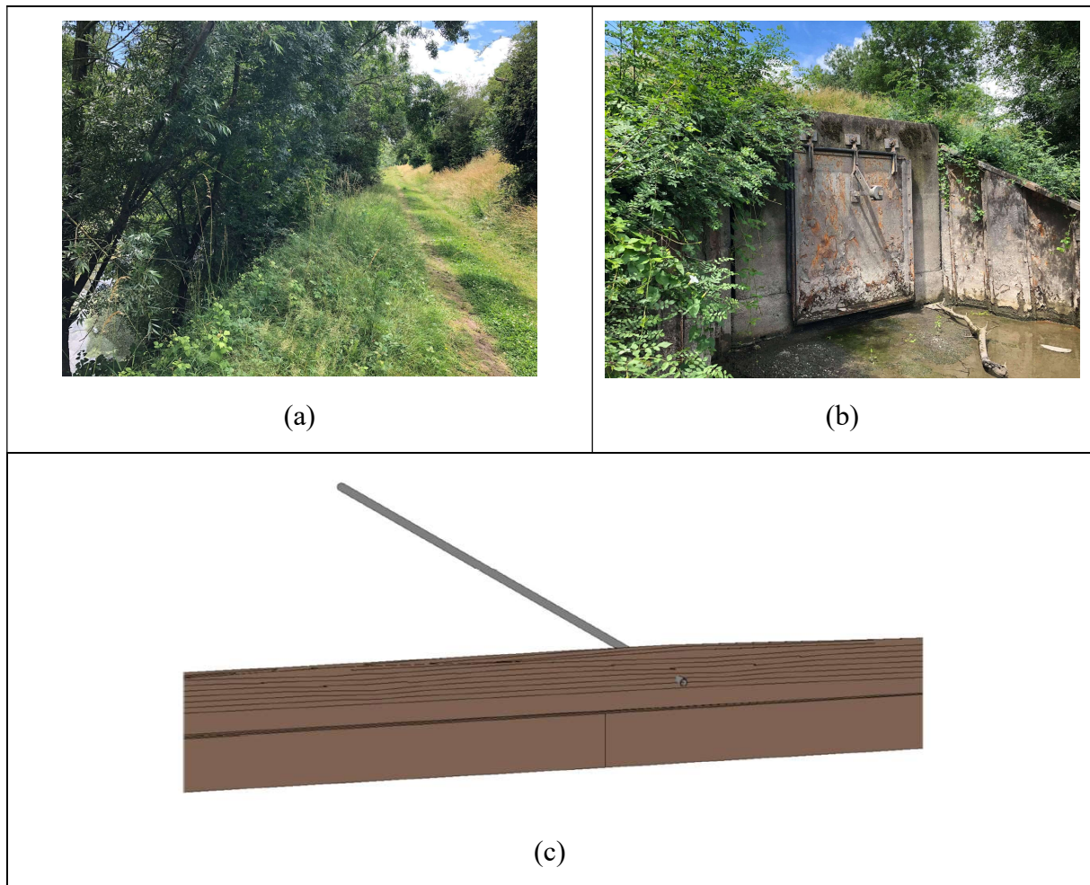
Fig. 7 : (a) vue d'une partie de la digue – (b) présence d'un ouvrage d'évacuation des eaux pluviales – (c) représentation de la digue et de l'ouvrage d'évacuation des eaux pluviales
