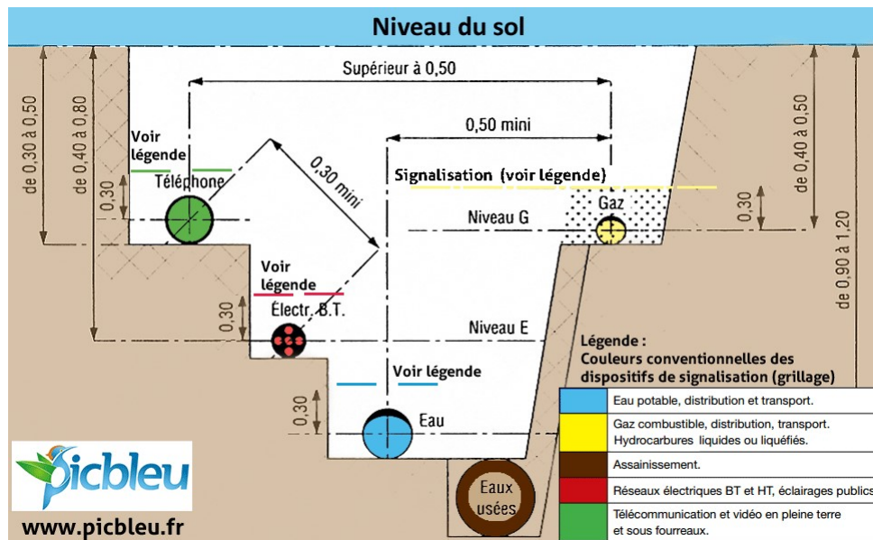
Fig. 8 : Distances minimales normalisées entre les différents types de réseaux – Source : Picbleu.fr
