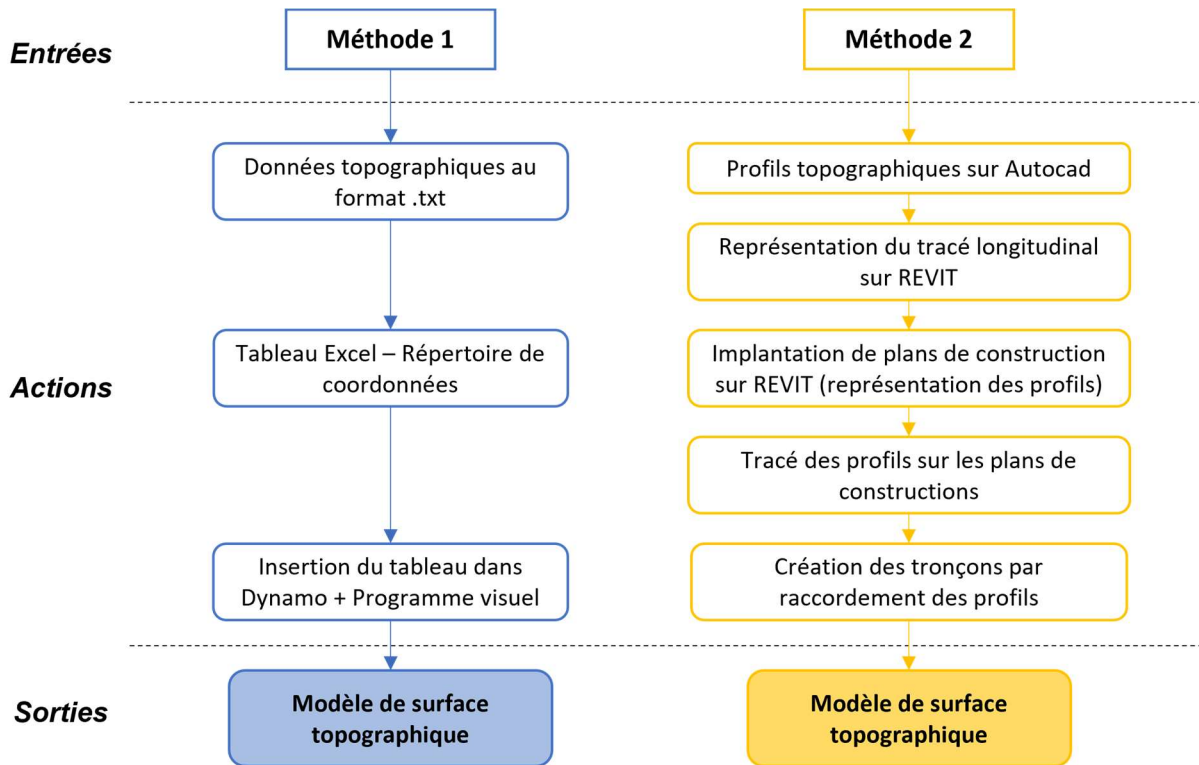
Fig. 2 : Logigramme des deux méthodes de modélisation de la digue
