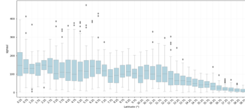
Fig. 13 Scale parameter ( \sigma ) by latitude
