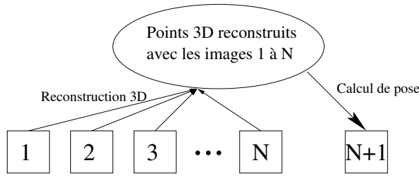
FIG. 2 – Calcul d’une solution initiale pour la pose de la caméra N+1
