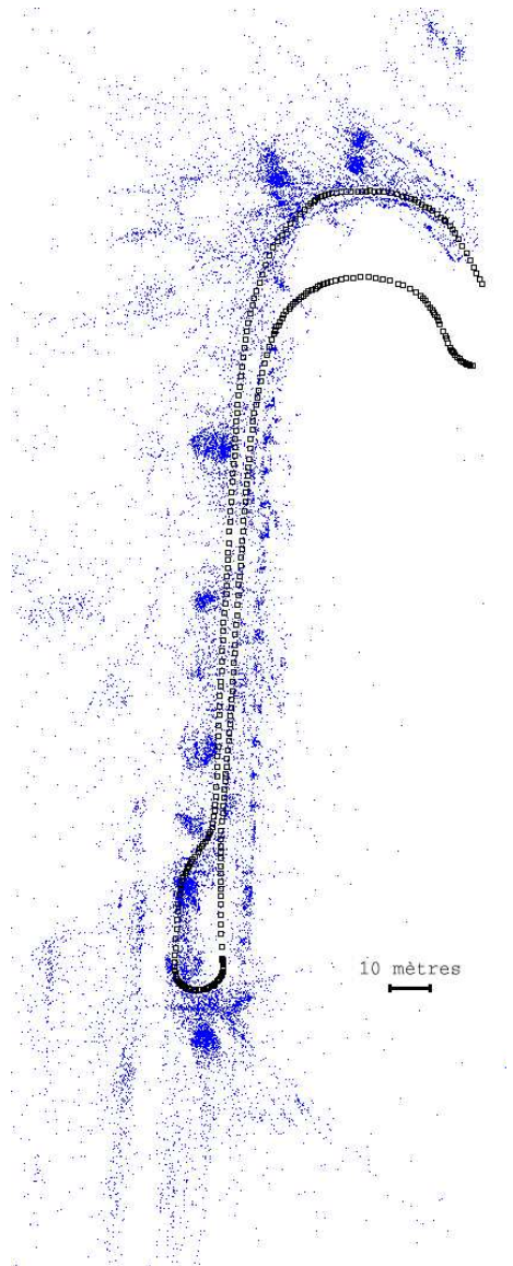
FIG. 16 – Reconstruction 3D d'une séquence de 400 m de long en aller-retour
