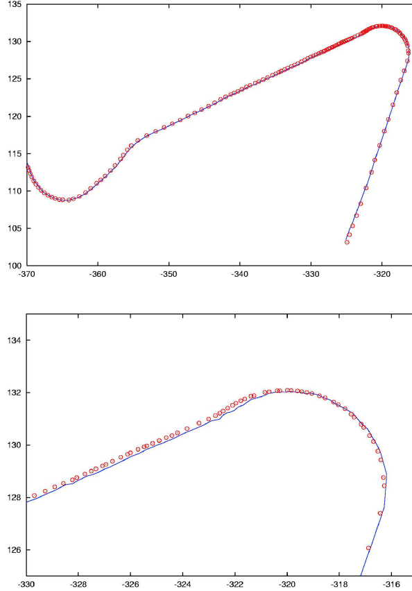
FIG. 7 – Position des images clef (cercles rouges) superposées à la trajectoire enregistrée par le GPS (ligne continue bleue), unités en mètres. La trajectoire complète est en haut et un agrandissement apparaît en bas
