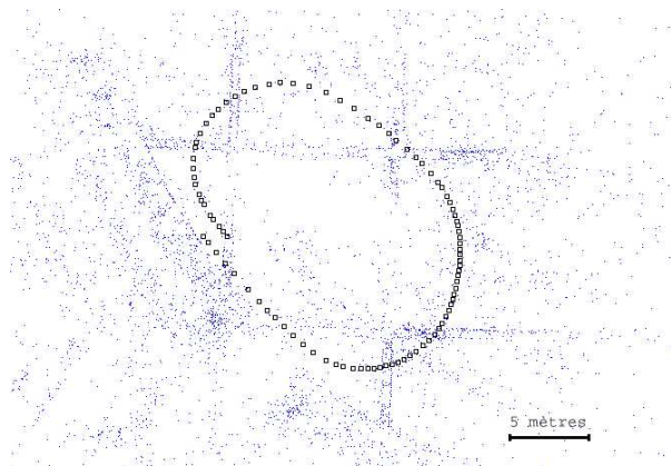
FIG. 10 – Reconstruction 3D d'une séquence en boucle
