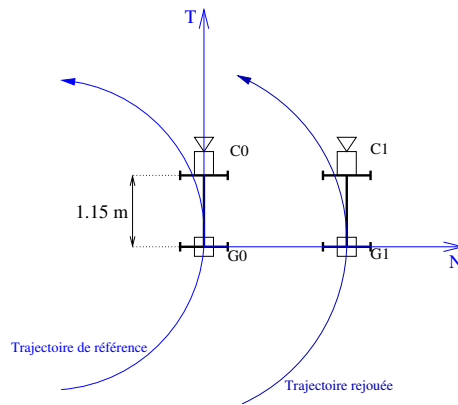
FIG. 8 – Calcul de l'écart latéral par rapport à la trajectoire de référence
