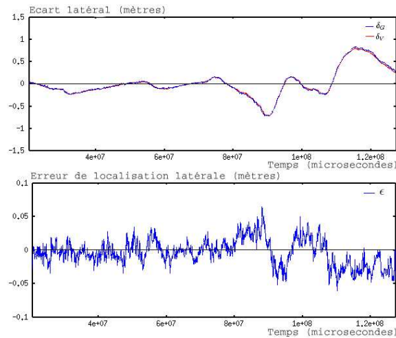
FIG. 9 – Erreur latérale (en haut) mesurée avec le GPS \delta_G (bleu) ou par vision \delta_V (rouge) et erreur de localisation latérale \epsilon (bas)
