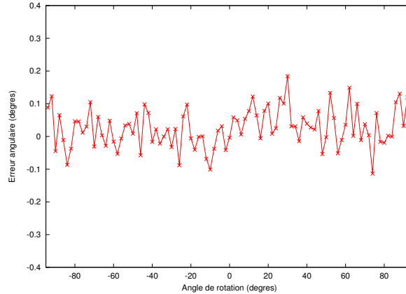
FIG. 14 – Erreur angulaire |\alpha_0| - |\alpha| en fonction de \alpha_0
