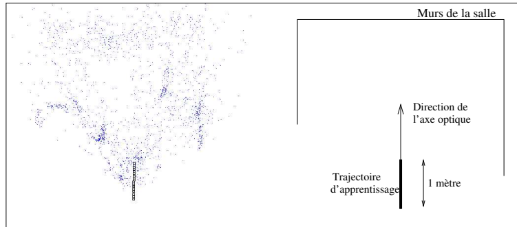
FIG. 13 – Reconstruction 3D utilisée pour évaluer la précision de l'orientation
