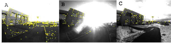
FIG. 4 – Appariement de points entre une image du flux vidéo (B et C) et l’image clef la plus proche (A). En B, soleil dans le champ de la caméra, en C, sol enneigé. Seuls les appariements corrects sont affichés.
