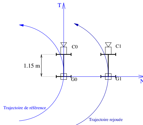
FIG. 8 – Calcul de l'écart latéral par rapport à la trajectoire de référence
