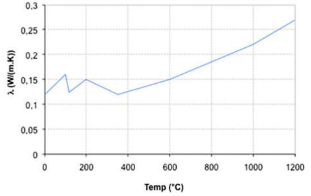
b) Thermal conductivity (Janssens)
