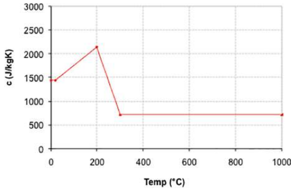
a) Specific heat (Fredlund / Janssens)
