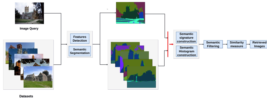
Fig. 2. Global framework
