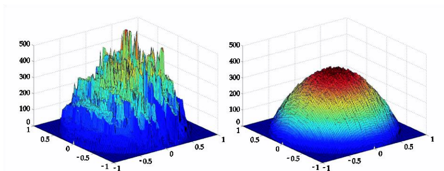
Figure 2. Visualisation des résultats en 3 dimensions d’une résolution d’équations aux dérivées partielles avec un mouvement brownien. A gauche avec la version standard du générateur rand sous Linux et à droite le résultat correct avec le générateur dit « Mersenne Twister ».
