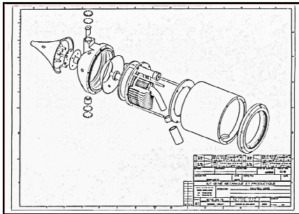
Fig.4 Plan d'ensemble.
