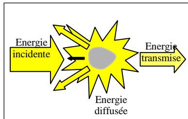
Fig.1 Phénomène de diffusion. Dans le cas de gouttes d'eau de diamètre supérieur à 100 \mu\text{m} une énergie importante est diffusée à environ 142^\circ : c'est l'arc en ciel. La flèche noir représente l'énergie rétrodiffusée utilisée dans le cas des radars et Lidar.
