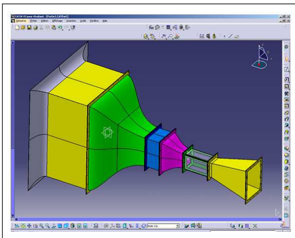
Fig.7 Plan d'ensemble sous CATIA de la première partie (convergent, petite veine de mesure).
