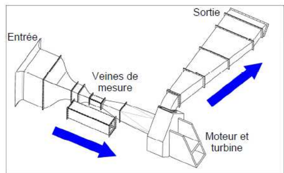
Fig.9 Vue d'ensemble de la soufflerie avec les 2 veines de mesure interchangeables.
