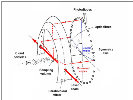
Fig.3 Principe de mesure du néphélomètre aéroporté.
