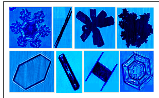
Fig.2 Différentes formes de cristaux de glace échantillonnés en nuage (étoile à 6 branches, aiguilles creuses, plaques hexagonales, particule givrée ...)
