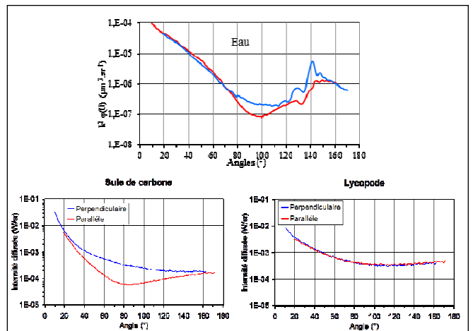
Fig.6 Différentes indicatrices de diffusion : l'énergie diffusée est représentée en fonction de l'angle. Dans le cas de l'eau on reconnaît les deux arcs en ciel. Le premier à environ 142^\circ et le deuxième, plus atténué, à 128^\circ . Si on fait tourner un polariseur devant son œil, à un moment donné l'arc en ciel disparaîtra car cette lumière diffusée est polarisée. Dans le cas du lycopode on a un aérosol très absorbant qui ne polarise pas la lumière diffusée.
